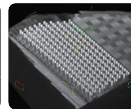
イメージセンサーの 極小TSV部の3Dモデル
