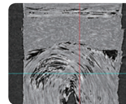
3Dプリンターで作成したCFRP積層 構造体断面像(繊維径:約7 \mu m)※
